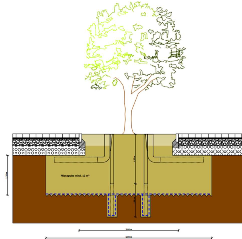
Längsschnitt Baumstandort
