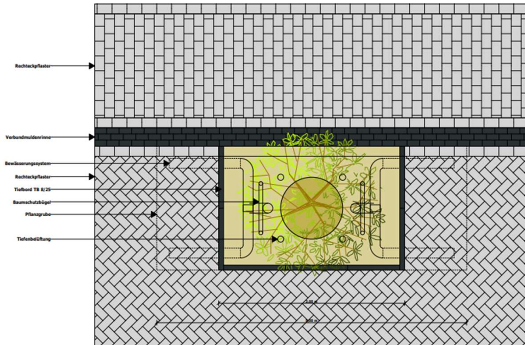
Draufsicht Baumstandort
