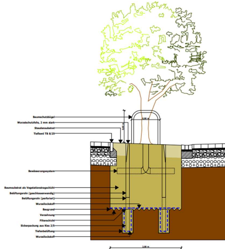
Querschnitt Baumstandort
